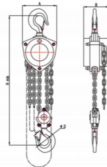
SLH-CSL 铝合金手拉葫芦 SLH-CSL aluminum alloy chain hoist
